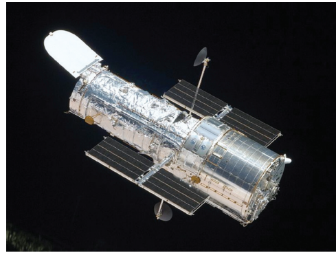
27- Foto do Telescópio Espacial Hubble feita pela tripulação do Space Shuttle Atlantis em maio de 2009, durante a quinta e última missão de reparo (crédito: NASA).
