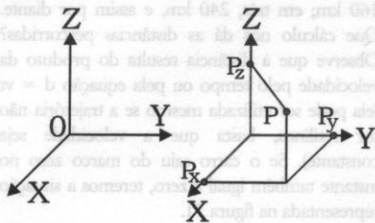
Figura 30 – Eixos cartesianos.
